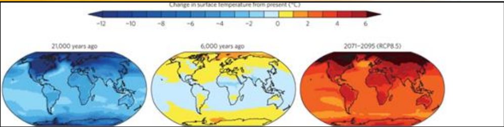
మోడల్-సిమ్యులేటెడ్ గ్లోబల్ టెంపరేచర్ అసాధారణతలు: లాస్ట్ హిమనదియ గరిష్ఠం (21,000 సంవత్సరాల క్రితం), మధ్య-హోలోసీన్ (6,000 సంవత్సరాల క్రితం), మరియు RCP8.5 కింద 2071-2095 కొరకు ప్రాజెక్షన్
